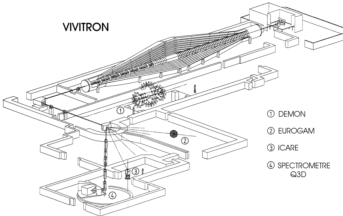
Figure II.12 : L'accélérateur VIVITRON et les aires expérimentales associées.
