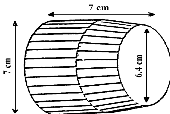
Figure II.16 : Représentation schématisée d'un détecteur Ge conique [DeF91].
