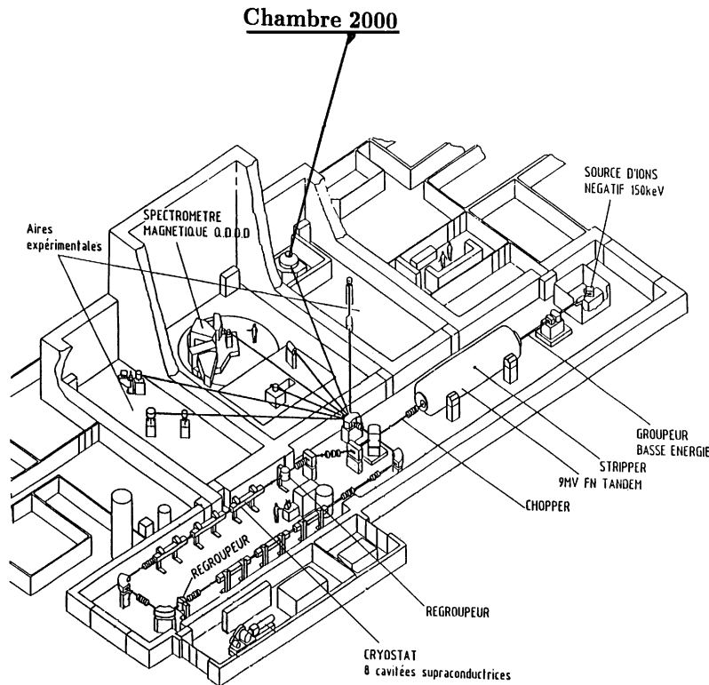
Figure II.5 : Tandem post-accéléré de Saclay (Schéma tiré de la référence [Val87]).
