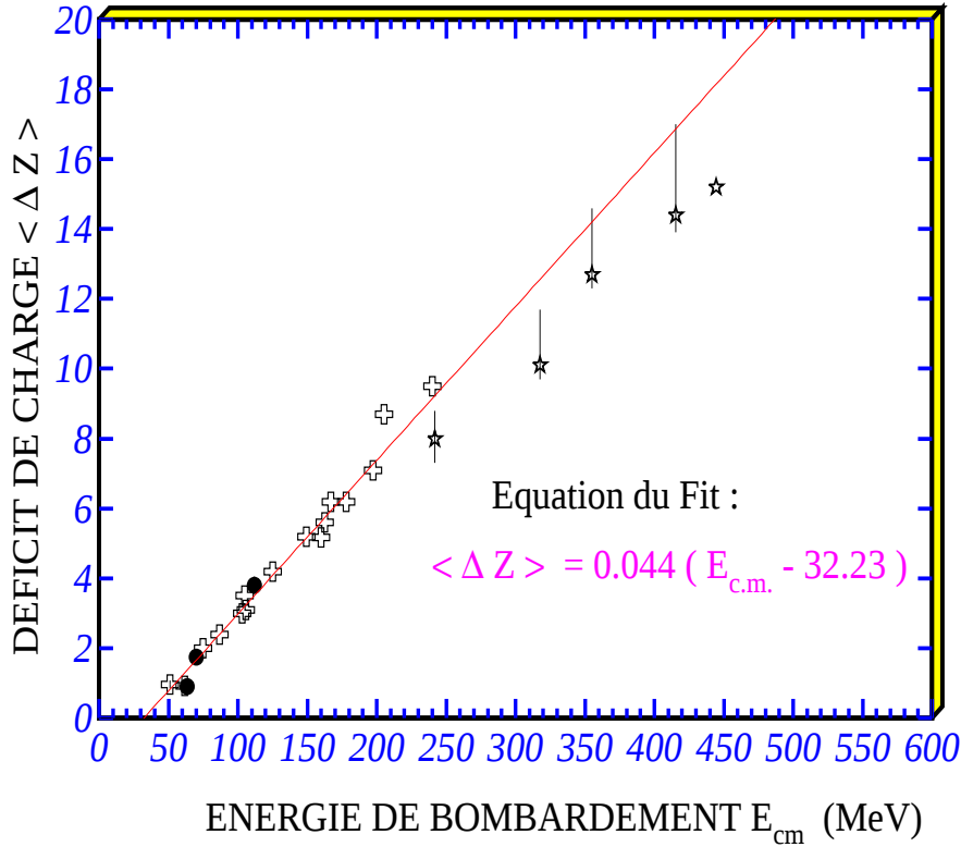
Figure III.22 : Systématique du déficit de charge nucléaire. La ligne continue représente le fit donnant l'équation de la systématique discutée dans le texte. Les étoiles représentent les données expérimentales pour des réactions au-dessus de 11 MeV/nucléon. Les croix représentent les données expérimentales pour des réactions en-dessous de 11 MeV/nucléon. Les points noirs représentent nos données expérimentales ^{35}\text{Cl} + ^{12}\text{C} et ^{35}\text{Cl} + ^{24}\text{Mg} .
