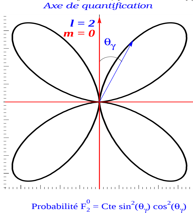
Figure III.49 : Schéma illustrant le comportement des distributions angulaires \gamma pour une transition quadrupolaire l = 2 et m = 0 .
