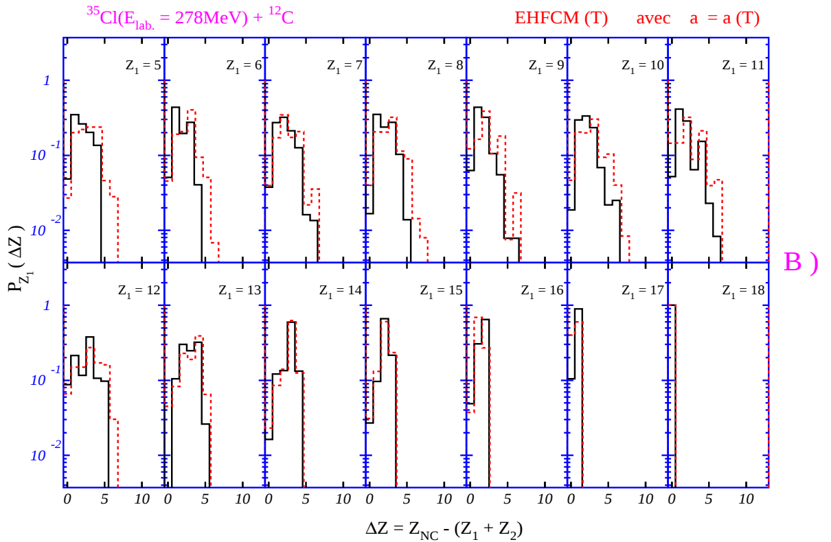
Figure IV.8 : Comparaison des distributions du déficit de charge des fragments Z_{1,2} \geq 5 en coïncidence mesurées pour la réaction ^{35}\text{Cl} + ^{12}\text{C} (histogramme en trait continu) aux calculs du modèle Hauser-Feshbach étendu (histogramme en trait discontinu)
