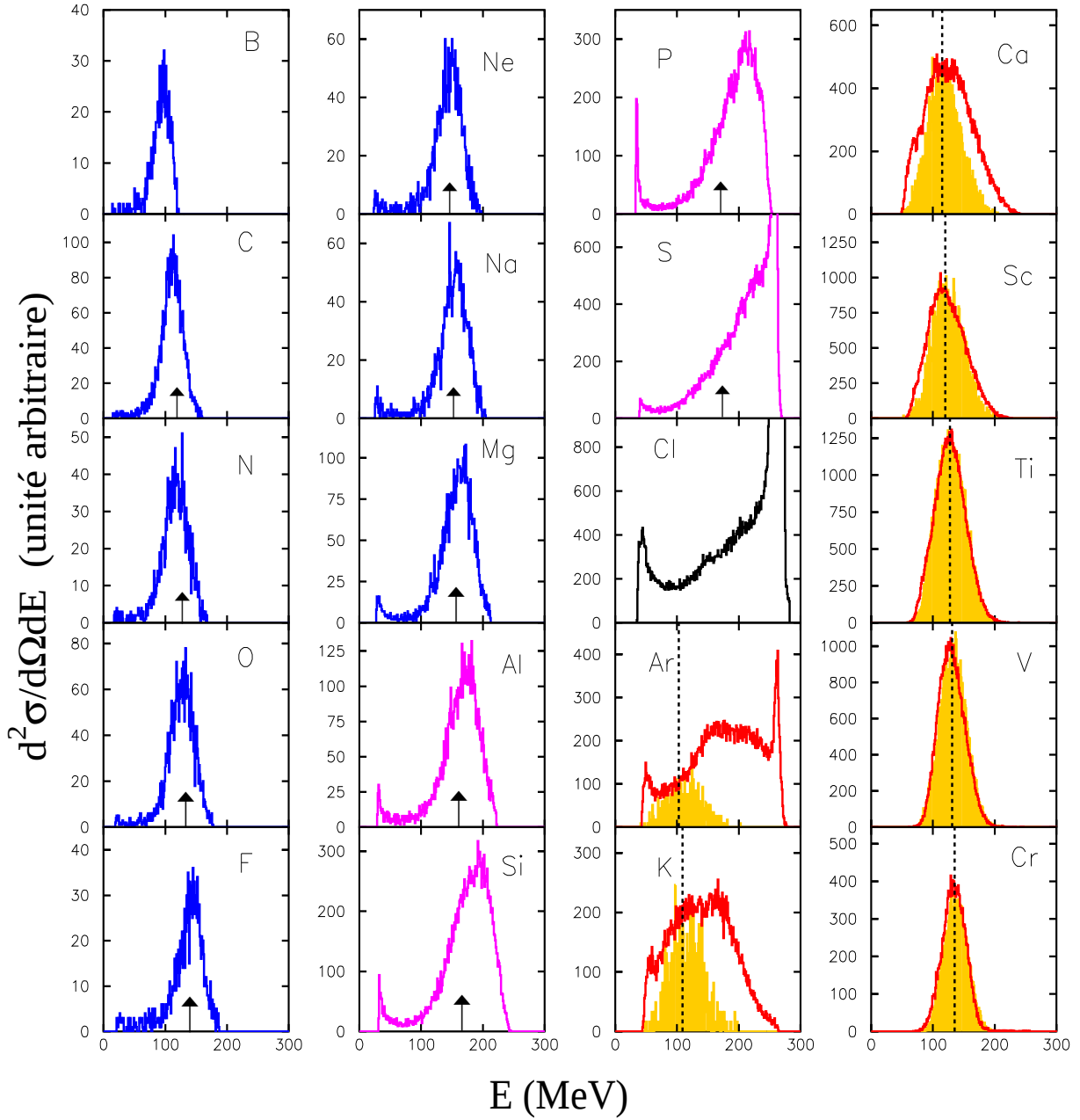
Figure III.2 : Spectres d'énergie expérimentaux (histogrammes vides) des fragments de charge 5 \leq Z \leq 24 issus de la réaction ^{35}\text{Cl} ( E_{\text{lab.}} = 275 \text{ MeV} ) + ^{24}\text{Mg} à \theta_{\text{lab.}} = -7^\circ . Les histogrammes pleins sont le résultat d'un calcul d'évaporation (LILITA). La flèche indique l'énergie attendue dans l'hypothèse d'une fragmentation binaire. La ligne discontinue correspond à l'énergie attendue dans l'hypothèse où le fragment est un résidu d'évaporation (voir le texte).
