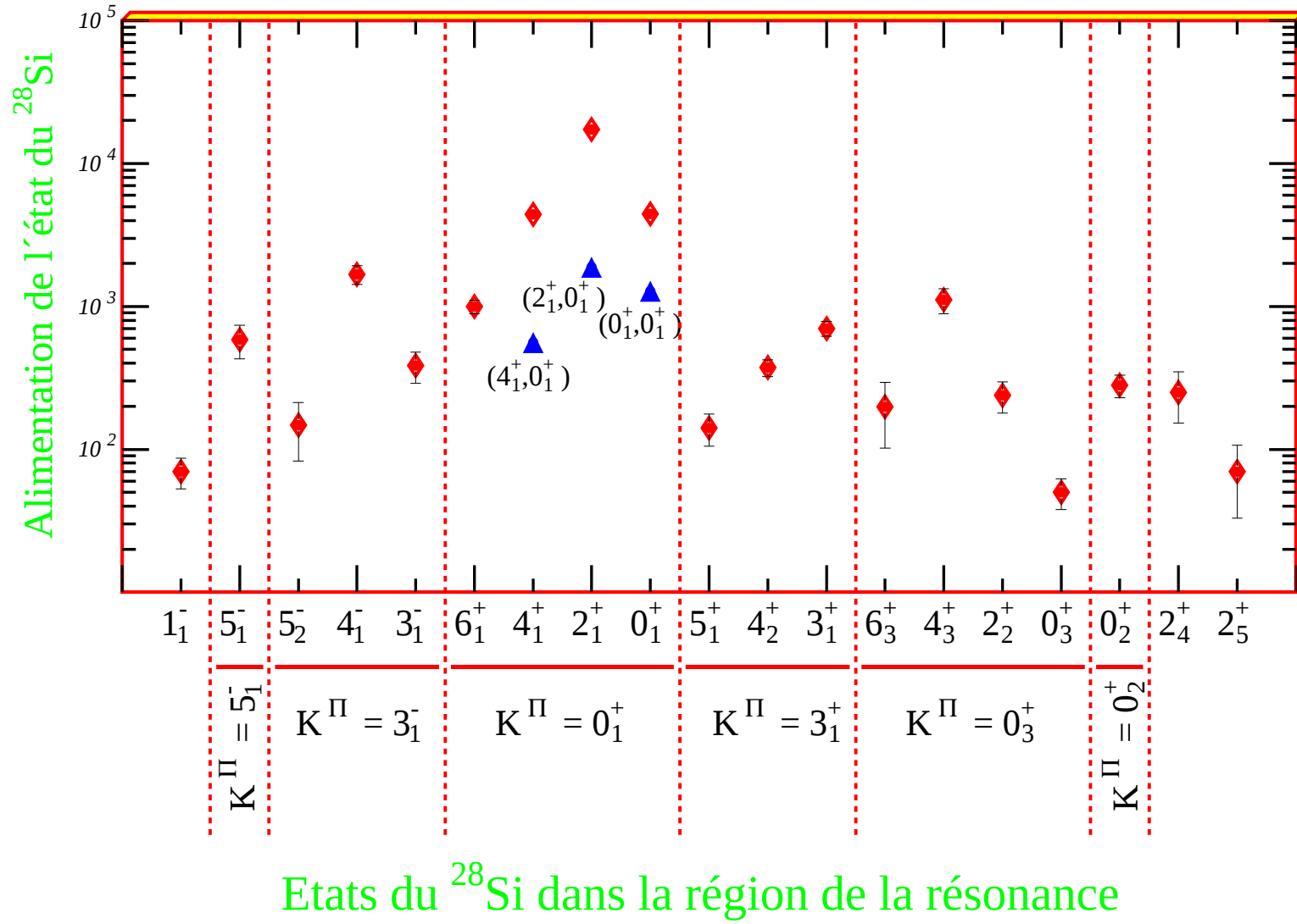
Figure III.44 : Alimentations des états du ^{28}\text{Si} obtenues en sélectionnant le domaine angulaire de la résonance 73.2^\circ \leq \theta_{cm} \leq 105.6^\circ lors de la réaction induite ^{28}\text{Si} + ^{28}\text{Si} à une énergie de résonance 111.6 MeV. Les points “Diamants rouges” correspondent à l'alimentation des états mutuels excités. Les points “Triangles bleus” correspondent à l'alimentation des états d'excitation simple.
