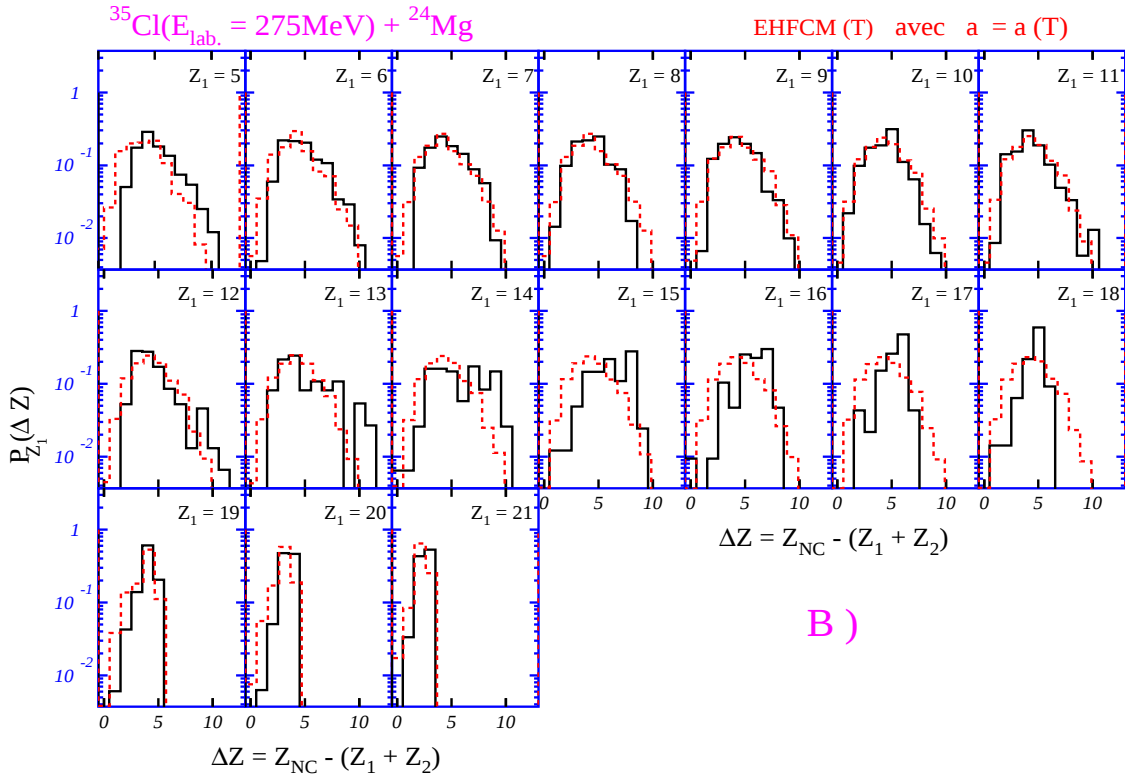
Figure IV.7 : Comparaison des distributions du déficit de charge des fragments Z_{1,2} \geq 5 en coïncidence mesurées pour la réaction ^{35}\text{Cl} + ^{24}\text{Mg} (histogramme en trait continu) aux calculs du modèle Hauser-Feshbach étendu (histogramme en trait discontinu)
