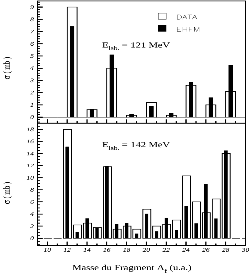
Figure II.2 : Distributions de masse expérimentales (histogrammes ouverts) pour la réaction ^{32}\text{S} + ^{24}\text{Mg} à E_{\text{lab.}} = 121 et 142 MeV [San89] comparés aux prédictions du modèle statistique Hauser-Feshbach Étendu (MEHF) (histogrammes pleins) [Mat97] (MEHF : voir chapitre IV).
