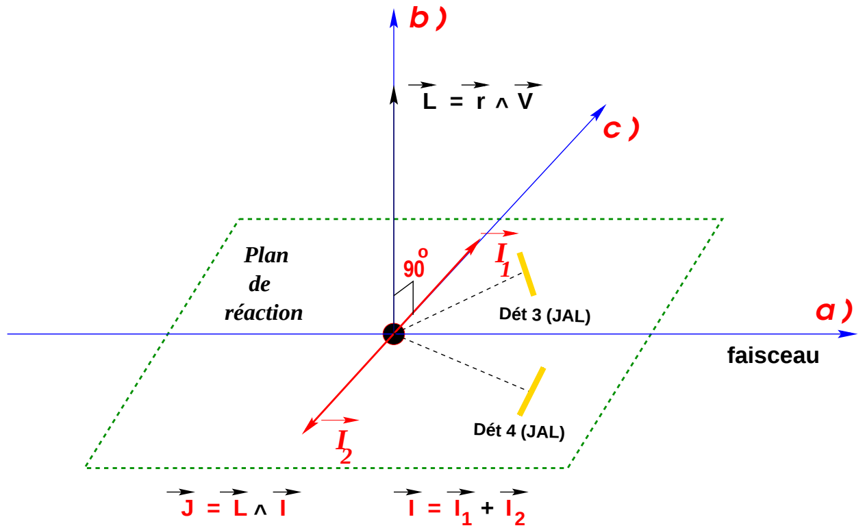
Figure III.48 : Schéma illustrant la direction des axes de quantification \vec{o}\hat{a} , \vec{o}\hat{b} et \vec{o}\hat{c} , la position des détecteurs de fragments (JAL) en coïncidence dans le plan de réaction par rapport aux axes de quantification. La direction du spin \vec{I} par rapport à la direction du moment orbital \vec{L} est illustré selon les indications données par les distributions angulaires \gamma présentées sur la figure III.47.
