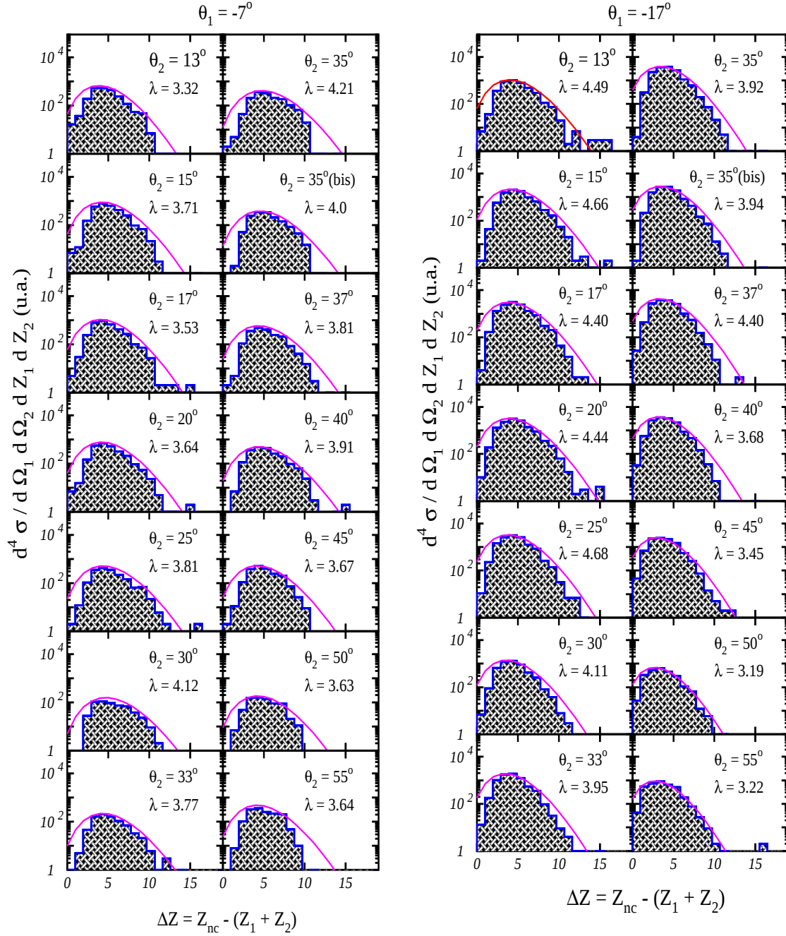
Figure III.20 : Distributions du déficit de charge \Delta Z mesurées à différentes configurations géométriques pour des fragments en coïncidence Z_{1,2} \geq 5 issus de la réaction ^{35}\text{Cl} + ^{24}\text{Mg} à E_{\text{lab.}} = 275 MeV. La courbe en continu correspond à un fit par une Poissonienne P(\Delta Z) = \mathcal{A} \lambda^{\Delta Z} e^{-\lambda} / \Delta Z! .
