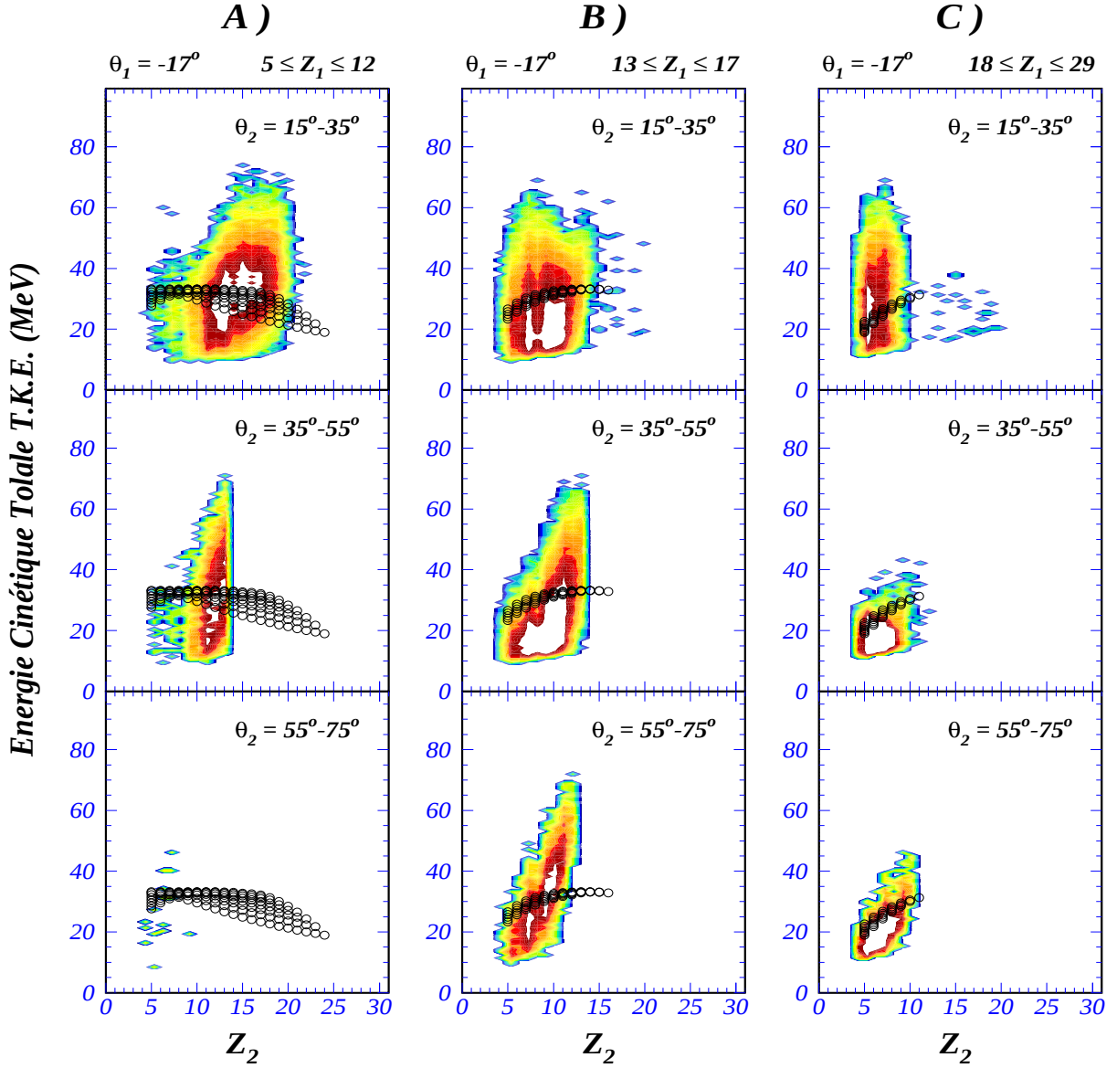
Figure III.28 : Spectres bidimensionnels T.K.E.- Z_2 pour la réaction ^{35}\text{Cl} + ^{24}\text{Mg} à E_{\text{lab}} = 275 \text{ MeV} . Les points (petits cercles) correspondent à l'énergie cinétique totale T.K.E. calculée dans le cadre d'un processus de fusion-fission symétrique et asymétrique discuté dans le texte.
