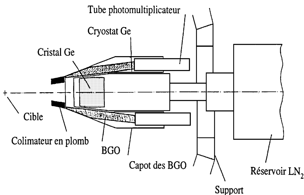
Figure II.17 : Coupe schématisée d'un détecteur Ge conique et de son enceinte anti-Compton de la phase II d'Eurogam [Bec92].
