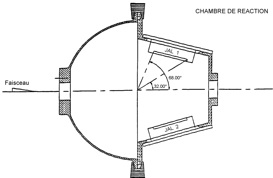
Figure II.13 : Schéma de la chambre à réaction utilisée pour l'expérience ^{28}\text{Si} + ^{28}\text{Si} .
