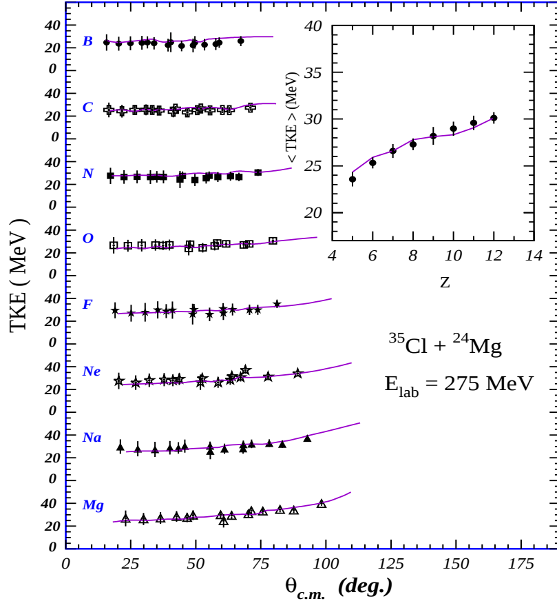
Figure IV.6 : Comparaison pour chaque élément 5 \leq Z \leq 12 des distributions angulaires de l'énergie cinétique totale T.K.E. des fragments de fusion-fission issus de la réaction ^{35}\text{Cl}(E_{\text{lab}} = 275 \text{ MeV}) + ^{24}\text{Mg} à celles calculées par la méthode de Hauser-Feshbach étendue avec calcul CASCADE indépendant de la température (courbe continue).
