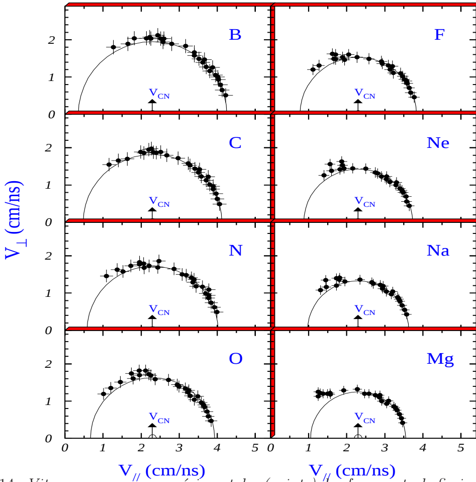
Figure III.14 : Vitesses moyennes expérimentales (points) des fragments de fission issus de la réaction ^{35}\text{Cl} ( E_{\text{lab.}} = 275 \text{ MeV} ) + ^{24}\text{Mg} représentés en fonction de ( V_{\parallel} , V_{\perp} ) par rapport à l'axe du faisceau. Les cercles ont été obtenus après lissage des données expérimentales.
