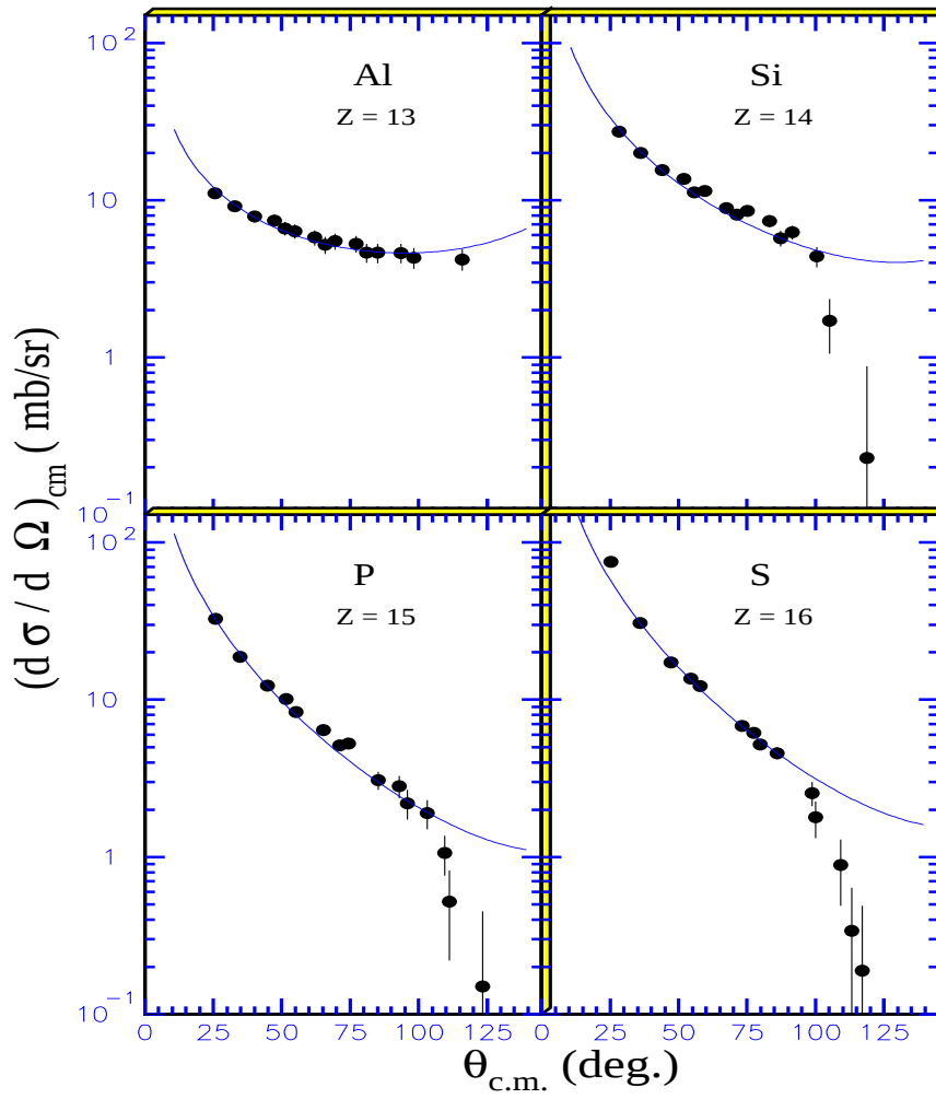
Figure III.13 : Distributions angulaires expérimentales (points) des produits binaires de charge 13 \leq Z \leq 16 issus de la réaction ^{35}\text{Cl} ( E_{\text{lab.}} = 275 \text{ MeV} ) + ^{24}\text{Mg} . La ligne continue correspond à un fit par d\sigma/d\Omega = (ae^{-\theta/\mu})/\sin(\theta) discuté dans le texte.
