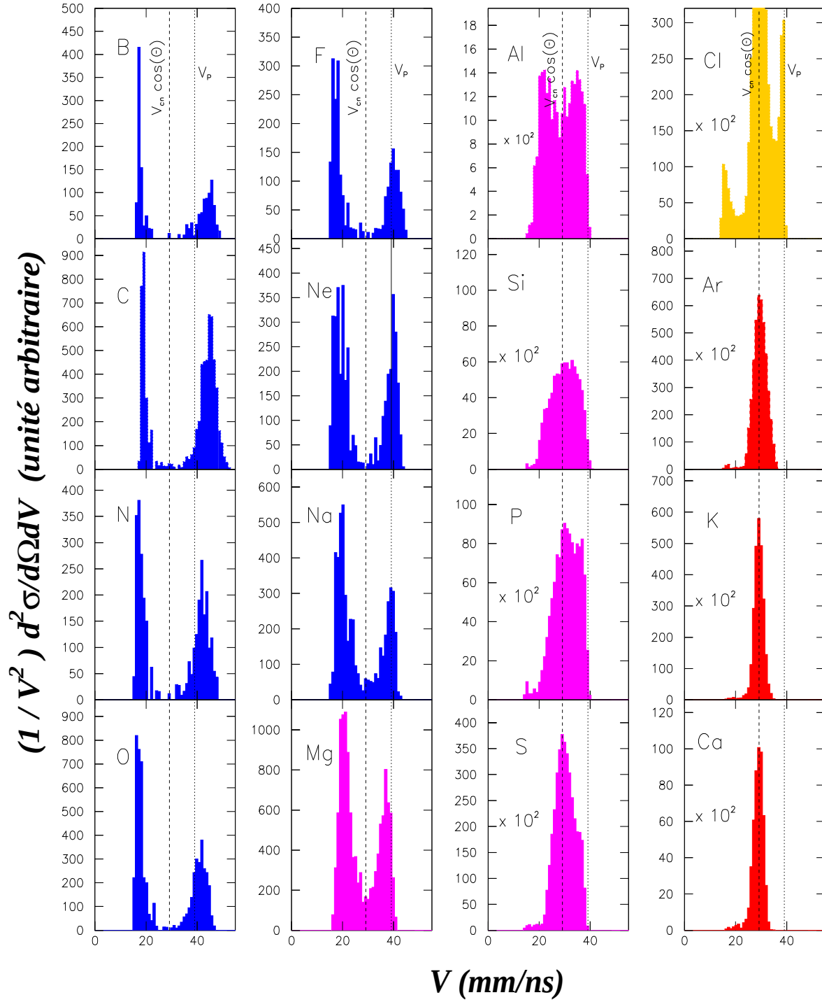
Figure III.6 : Spectres invariants de vitesse des fragments 5 \leq Z \leq 20 issus de la réaction ^{35}\text{Cl} ( E_{\text{lab.}} = 278 MeV) + ^{12}\text{C} à \theta_{\text{lab.}} = -7^\circ . La ligne en pointillé correspond à la vitesse du projectile V_p = 39.1 (mm/ns) et la ligne discontinue correspond à V_{nc} \cos(\theta) = 29.1 (mm/ns).
