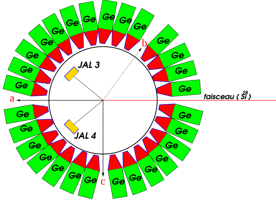
Figure III.46 : Schéma illustrant la disposition des différents axes de quantification \vec{oa} , \vec{ob} et \vec{oc}
