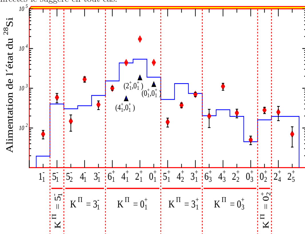
Etats du ^{28}\text{Si} dans la région de la résonance
