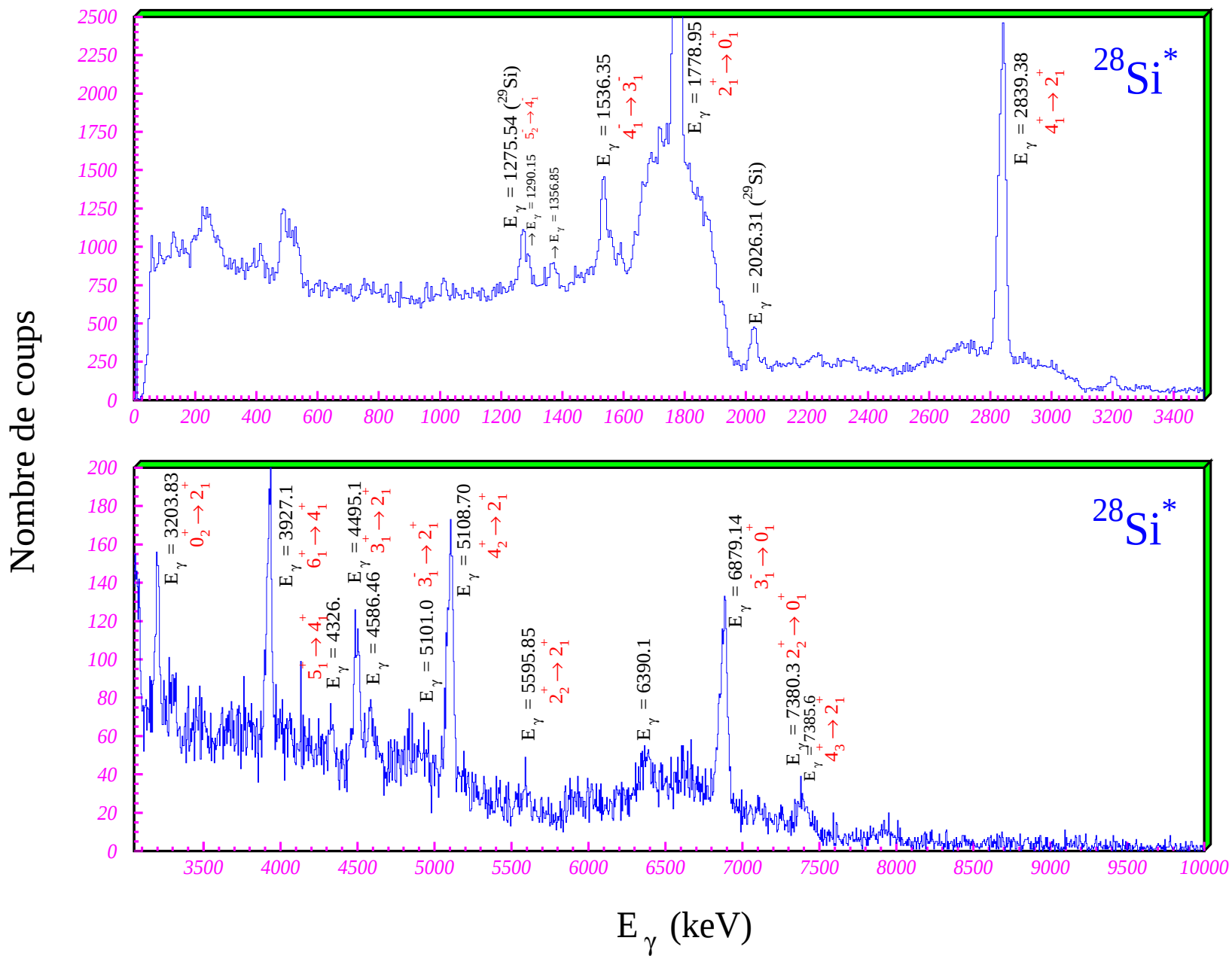
Figure III.38 : Spectre des rayonnements \gamma après correction Doppler émis en coïncidence avec un fragment ^{28}\text{Si} lors de la réaction ^{28}\text{Si} + ^{28}\text{Si} à une énergie de résonance 111.6 MeV. La subdivision du spectre en deux parties E_\gamma < 3500 keV et E_\gamma > 3000 keV permet plus de lisibilité.
