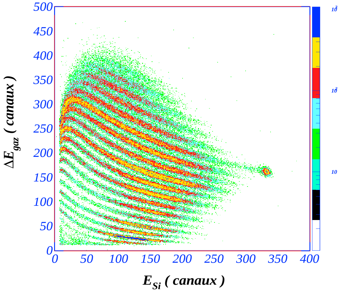
Figure II.8 : Exemple d'un spectre (E_{\text{Si}}, \Delta E_{\text{gaz}}) non calibré issu de la réaction ^{35}\text{Cl} + ^{24}\text{Mg}
