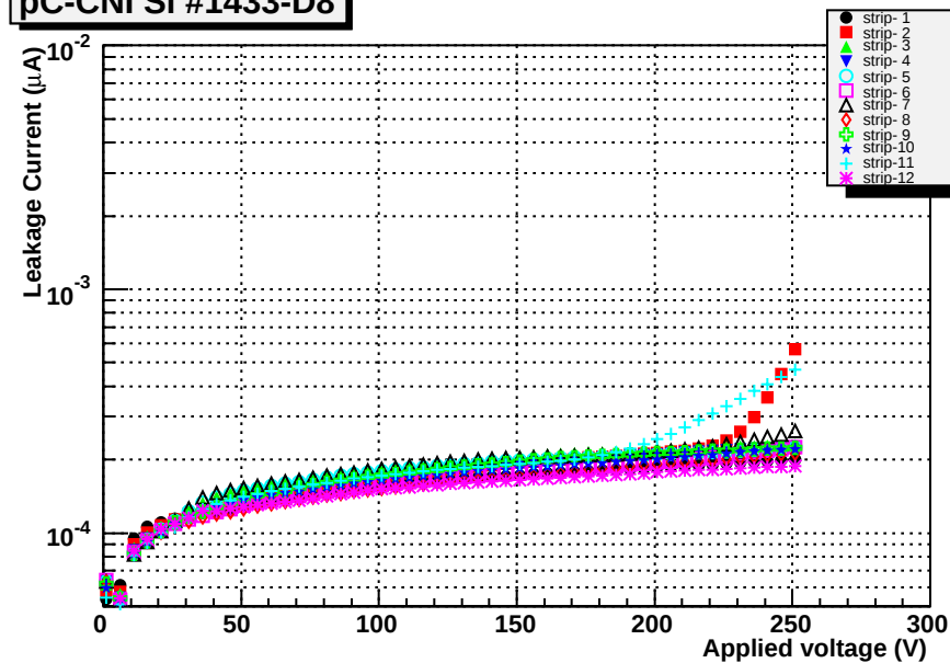
pC-CNI Si #1433-D8
