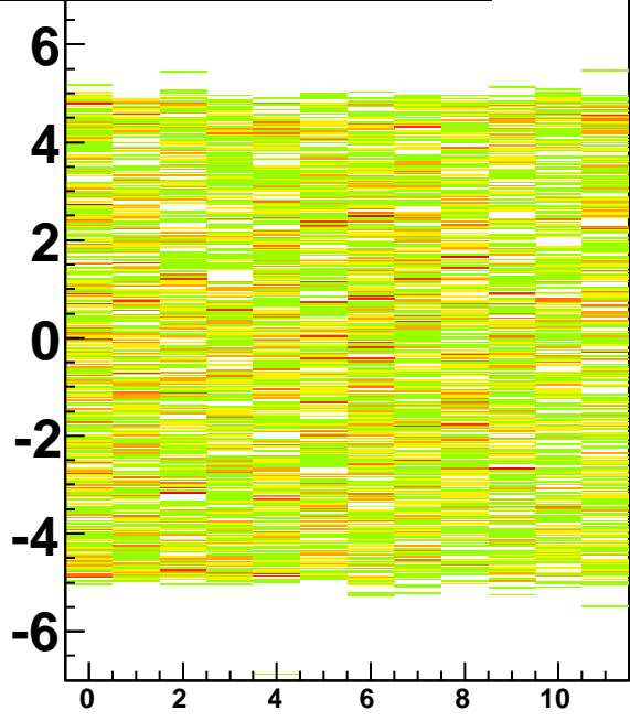
hmtdhitz_strip_zoff pos=4 BL30
