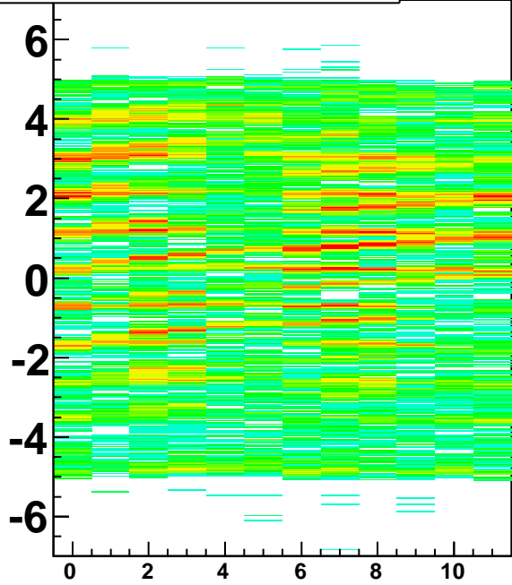
hmtdhitz_strip_zoff pos=5 BL30
