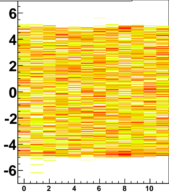
hmtdhitz_strip_zoff pos=3 BL30
