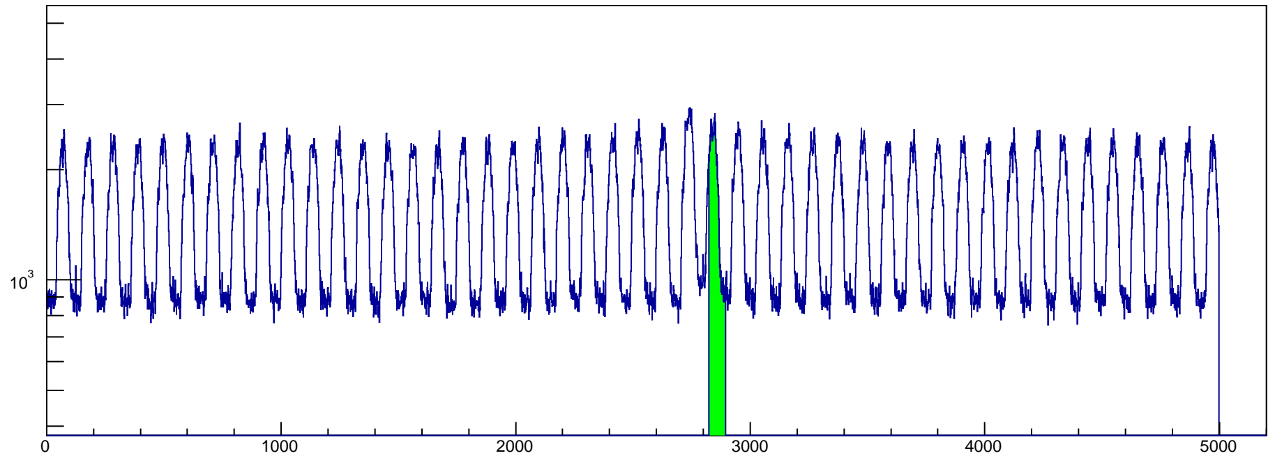
htrgdttime_mtd1
