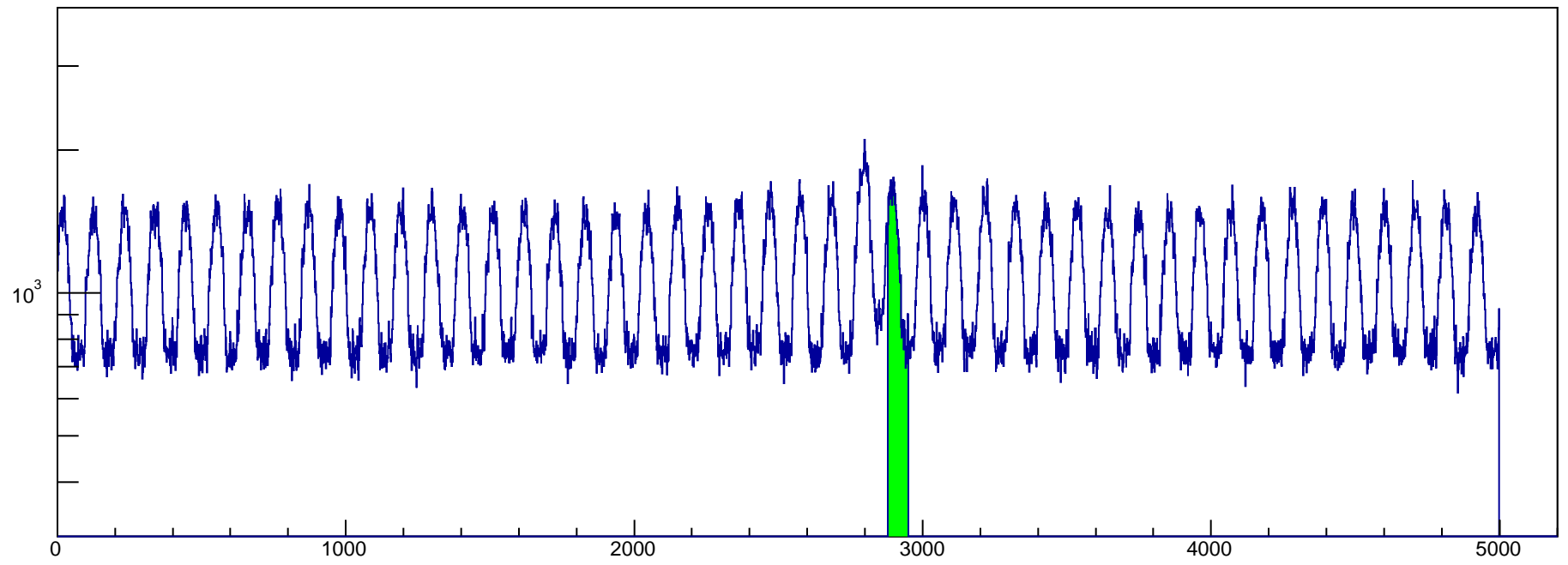
htrgdttime_mtd1
