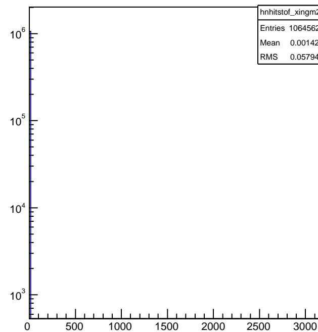
hnhitstof_xingm2
