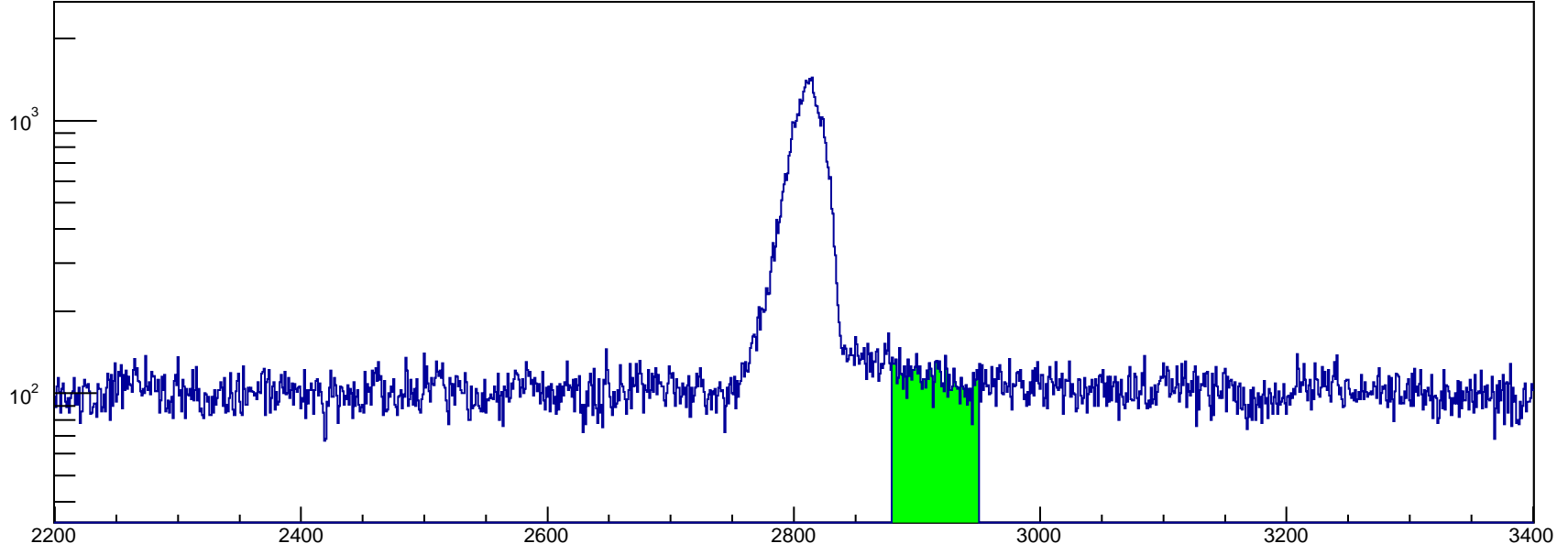
htrgdttime_mtd1
