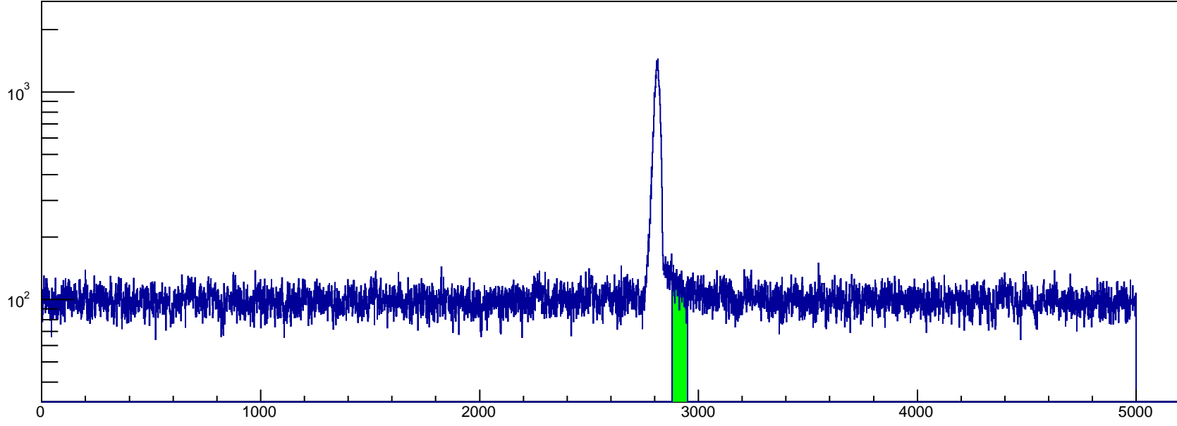
htrgdttime_mtd1
