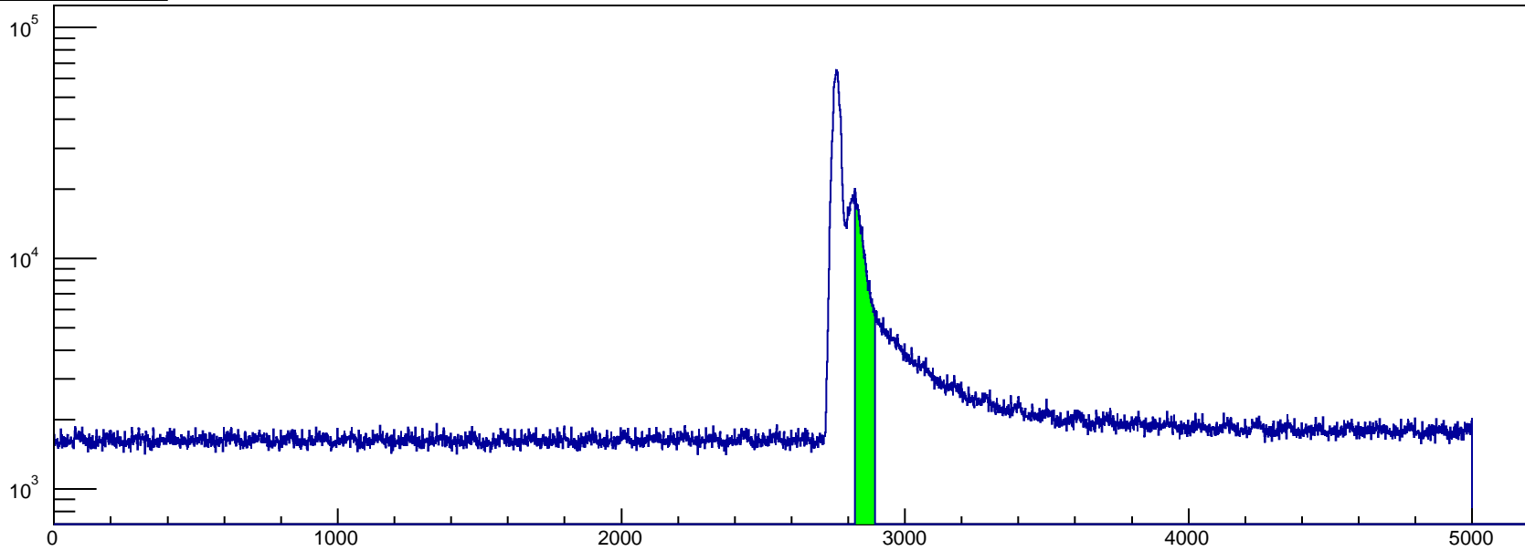
htrgdtime_mtd1
