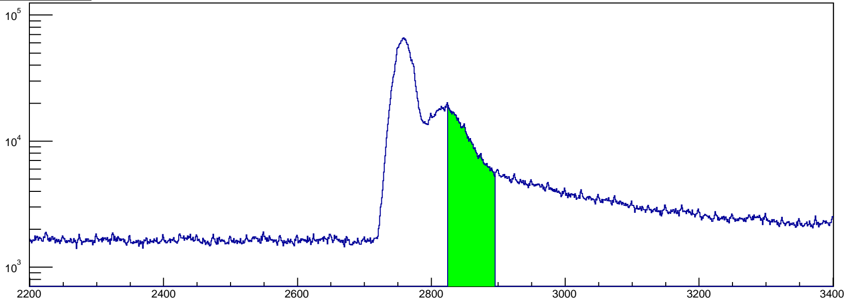
htrgdttime_mtd1
