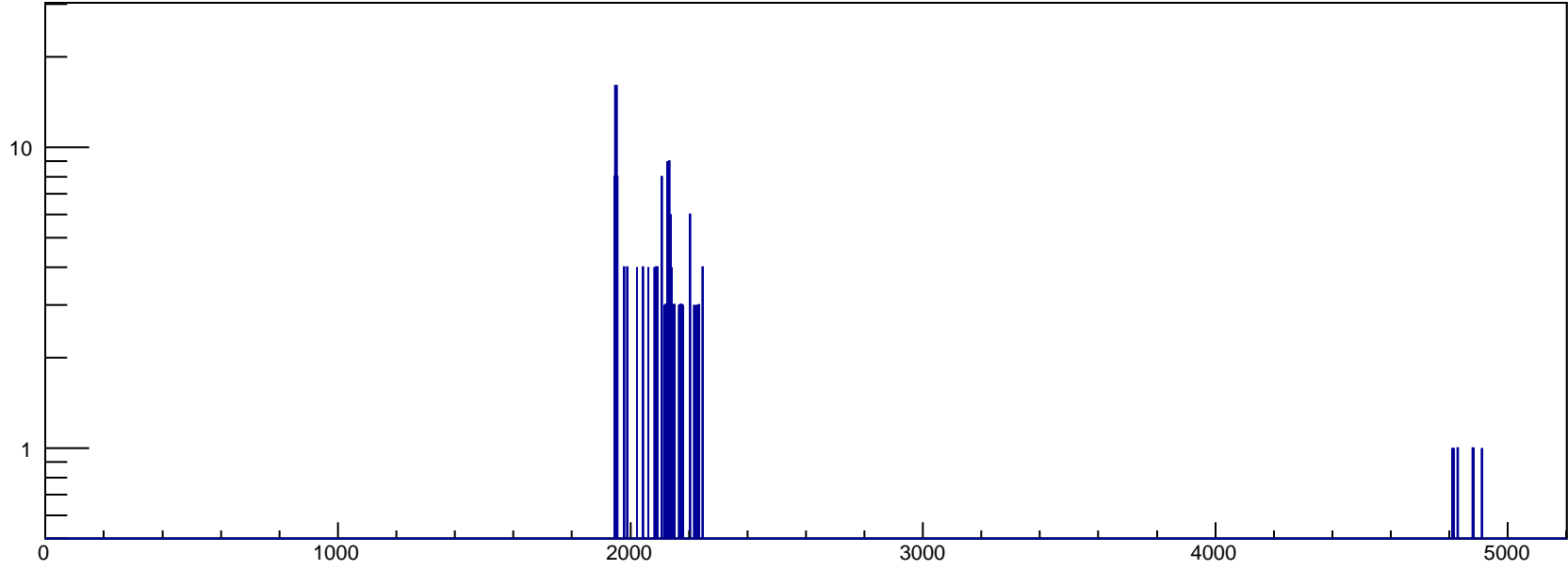
htrgdtime_mtd1
