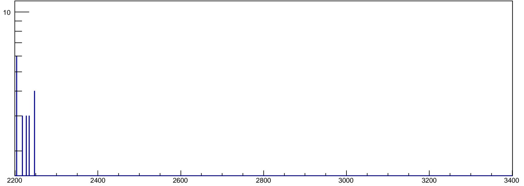
htrgdtime_mtd1
