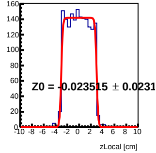
Module 5 Tray84 : z Local Fit
