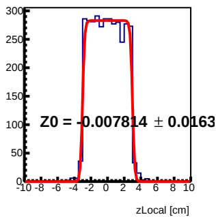
Module 3 Tray84 : z Local Fit
