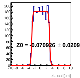
Module 4 Tray80 : z Local Fit
