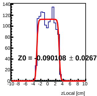
Module 5 Tray22 : z Local Fit
