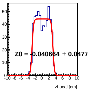
Module 2 Tray101 : z Local Fit
