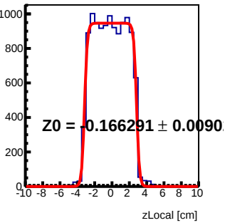
Module 6 Tray44 : z Local Fit
