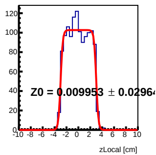
Module 1 Tray60 : z Local Fit
