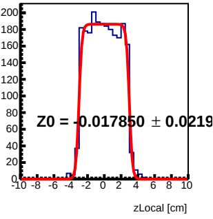
Module 4 Tray86 : z Local Fit
