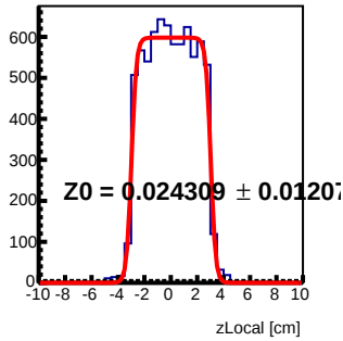
Module 6 Tray35 : z Local Fit
