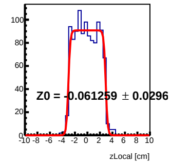
Module 5 Tray61 : z Local Fit
