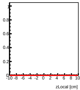
Module 5 Tray102 : z Local Fit
