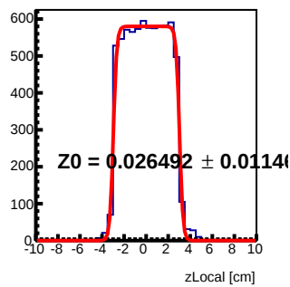
Module 6 Tray105 : z Local Fit
