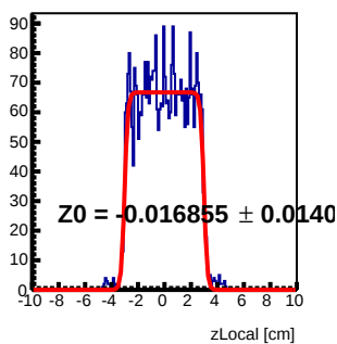
Module 4 Tray38 : z Local Fit
