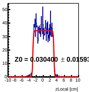
Module 5 Tray94 : z Local Fit
