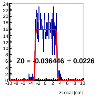
Module 2 Tray37 : z Local Fit
