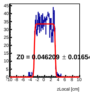
Module 5 Tray88 : z Local Fit
