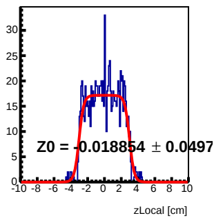
Module 2 Tray28 : z Local Fit
