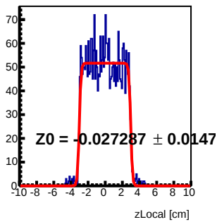
Module 4 Tray61 : z Local Fit
