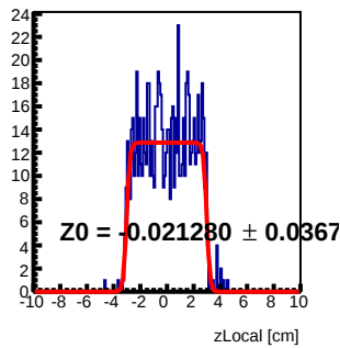
Module 2 Tray41 : z Local Fit
