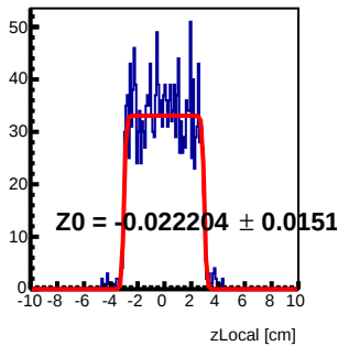
Module 5 Tray14 : z Local Fit
