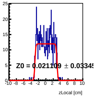
Module 2 Tray40 : z Local Fit
