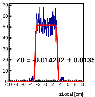
Module 4 Tray30 : z Local Fit
