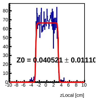
Module 4 Tray87 : z Local Fit
