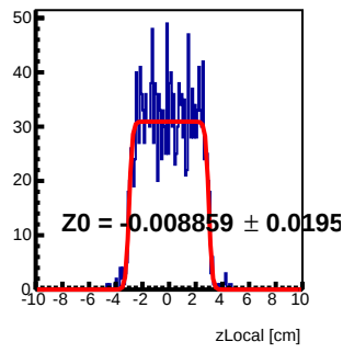
Module 5 Tray67 : z Local Fit
