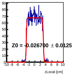
Module 4 Tray57 : z Local Fit
