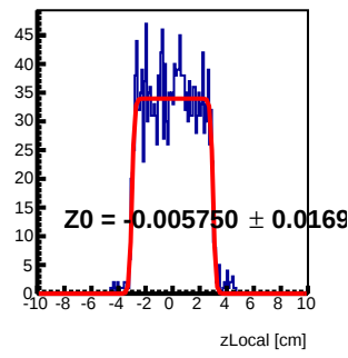
Module 5 Tray68 : z Local Fit
