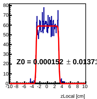
Module 4 Tray41 : z Local Fit
