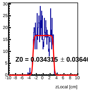
Module 2 Tray29 : z Local Fit
