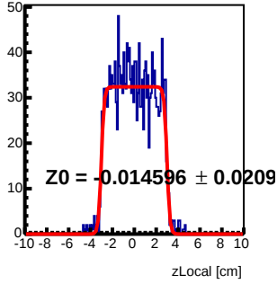
Module 5 Tray74 : z Local Fit
