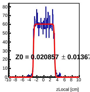
Module 4 Tray26 : z Local Fit
