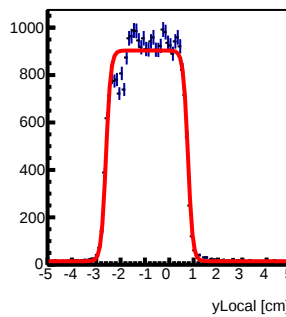
Tray107 : y Local Fit
