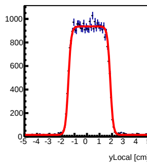
Tray119 : y Local Fit
