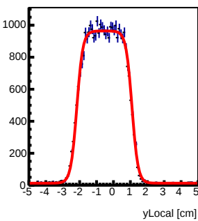
Tray38 : y Local Fit
