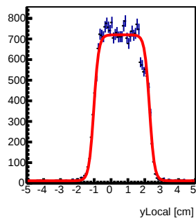
Tray5 : y Local Fit
