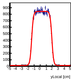
Tray1 : y Local Fit
