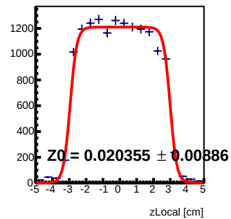
Module 0 Tray64 : z Local Fit
