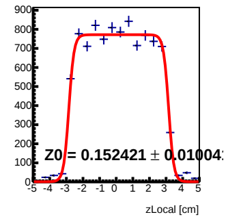
Module 4 Tray4 : z Local Fit
