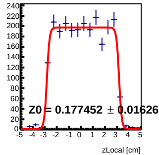
Module 2 Tray73 : z Local Fit
