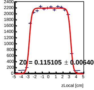
Module 6 Tray117 : z Local Fit
