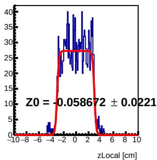
Module 0 Tray37 : z Local Fit
