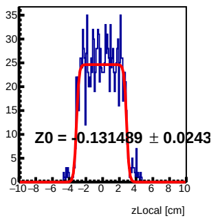
Module 3 Tray108 : z Local Fit
