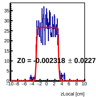
Module 0 Tray24 : z Local Fit
