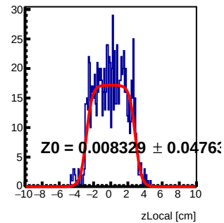
Module 3 Tray55 : z Local Fit
