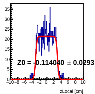
Module 3 Tray63 : z Local Fit
