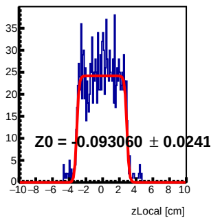
Module 3 Tray112 : z Local Fit
