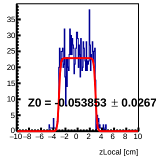
Module 0 Tray32 : z Local Fit
