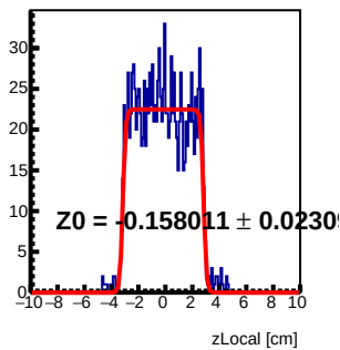
Module 3 Tray104 : z Local Fit
