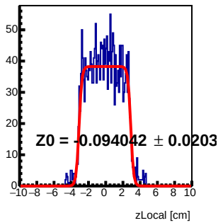
Module 6 Tray71 : z Local Fit
