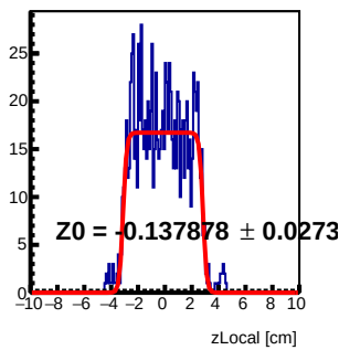
Module 3 Tray116 : z Local Fit
