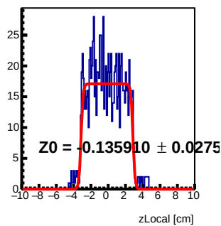
Module 3 Tray46 : z Local Fit
