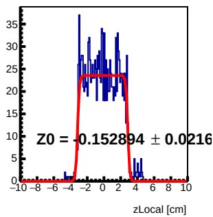
Module 3 Tray69 : z Local Fit
