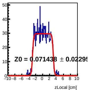
Module 0 Tray13 : z Local Fit
