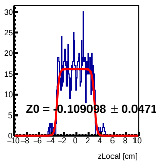
Module 3 Tray120 : z Local Fit
