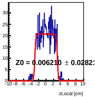
Module 0 Tray5 : z Local Fit
