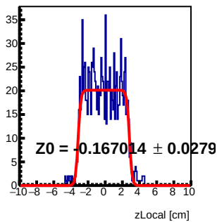
Module 3 Tray84 : z Local Fit
