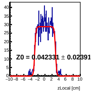
Module 0 Tray12 : z Local Fit
