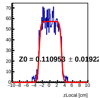
Module 6 Tray14 : z Local Fit
