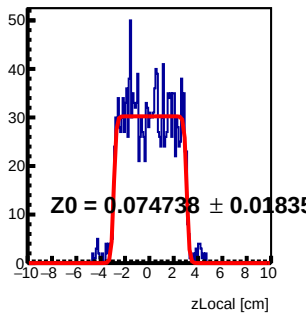
Module 0 Tray113 : z Local Fit
