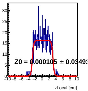
Module 3 Tray76 : z Local Fit
