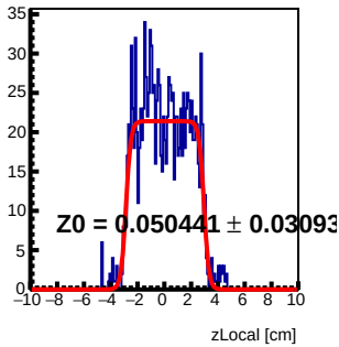
Module 0 Tray6 : z Local Fit
