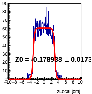
Module 6 Tray43 : z Local Fit
