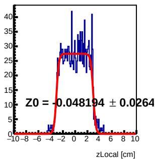
Module 0 Tray33 : z Local Fit
