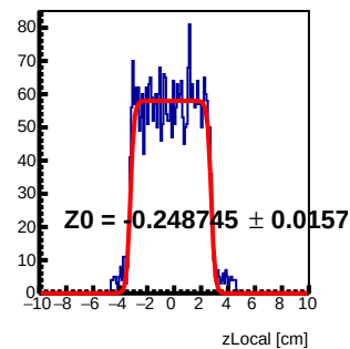
Module 6 Tray34 : z Local Fit
