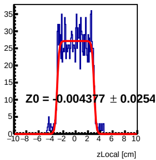
Module 0 Tray117 : z Local Fit
