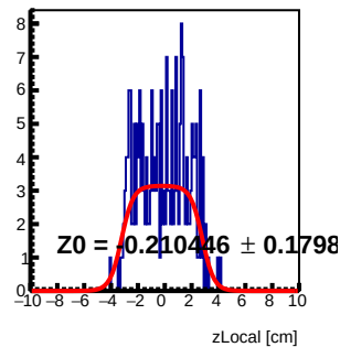
Module 2 Tray25 : z Local Fit
