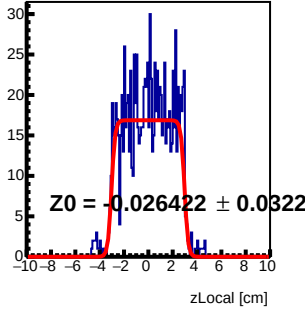
Module 0 Tray65 : z Local Fit
