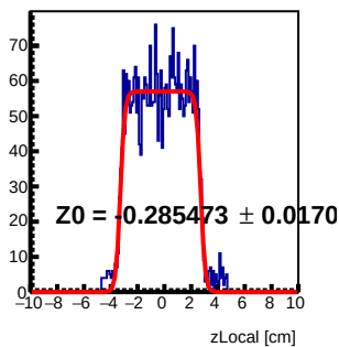
Module 6 Tray39 : z Local Fit
