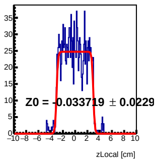
Module 3 Tray48 : z Local Fit
