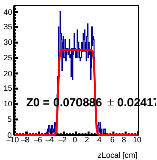
Module 0 Tray18 : z Local Fit
