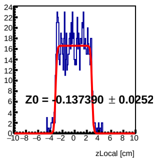
Module 3 Tray40 : z Local Fit
