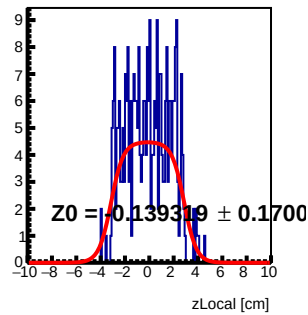
Module 2 Tray48 : z Local Fit
