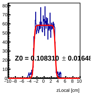
Module 6 Tray19 : z Local Fit
