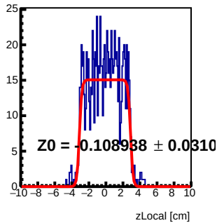
Module 3 Tray65 : z Local Fit
