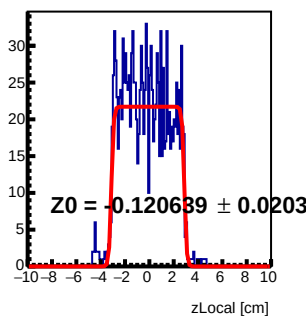
Module 3 Tray32 : z Local Fit
