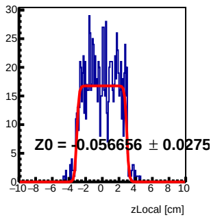
Module 3 Tray80 : z Local Fit
