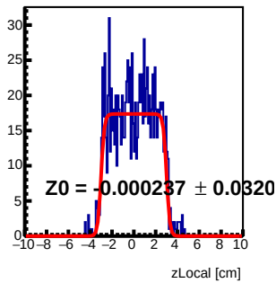
Module 0 Tray105 : z Local Fit
