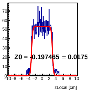
Module 6 Tray119 : z Local Fit
