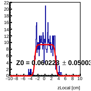
Module 0 Tray8 : z Local Fit
