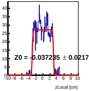
Module 0 Tray73 : z Local Fit
