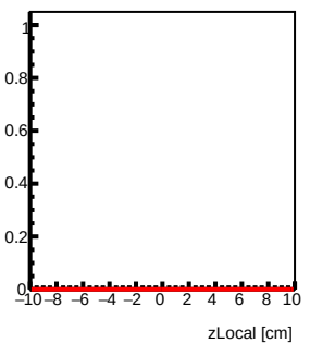
Module 6 Tray103 : z Local Fit
