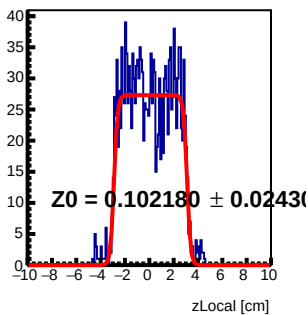
Module 0 Tray14 : z Local Fit
