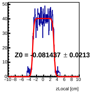
Module 6 Tray111 : z Local Fit
