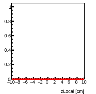
Module 6 Tray22 : z Local Fit
