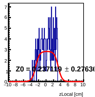
Module 2 Tray56 : z Local Fit
