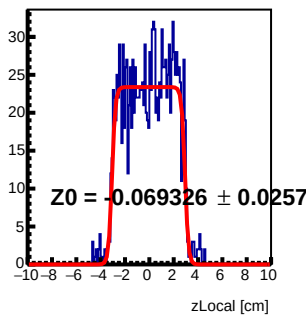
Module 3 Tray72 : z Local Fit
