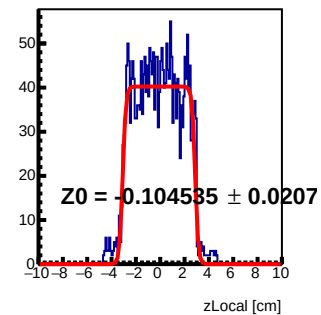
Module 6 Tray10 : z Local Fit
