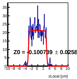
Module 4 Tray43 : z Local Fit
