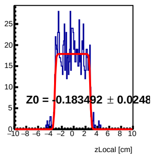
Module 3 Tray26 : z Local Fit
