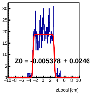
Module 0 Tray21 : z Local Fit
