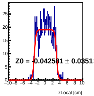
Module 0 Tray25 : z Local Fit
