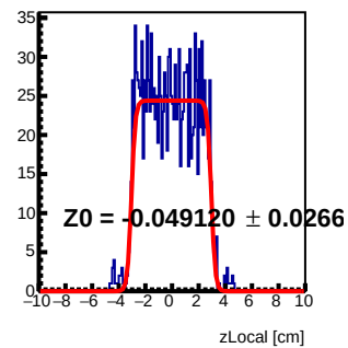
Module 3 Tray47 : z Local Fit
