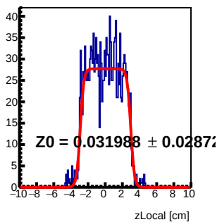
Module 0 Tray17 : z Local Fit
