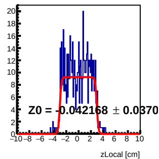
Module 0 Tray96 : z Local Fit
