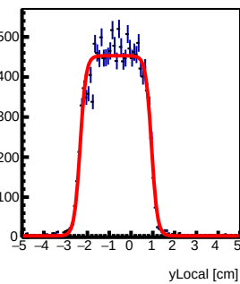
Tray46 : y Local Fit
