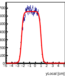
Tray42 : y Local Fit
