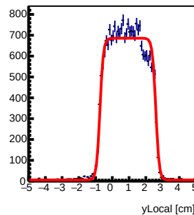
Tray19 : y Local Fit
