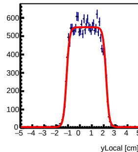
Tray11 : y Local Fit
