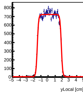
Tray7 : y Local Fit
