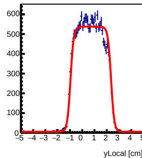
Tray15 : y Local Fit
