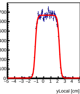
Tray22 : y Local Fit
