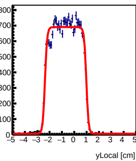
Tray54 : y Local Fit
