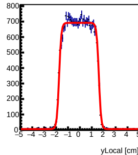
Tray3 : y Local Fit
