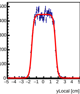
Tray30 : y Local Fit
