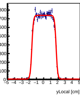
Tray58 : y Local Fit
