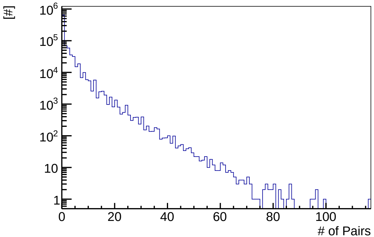
Step 6 : # of Valid Pairs
