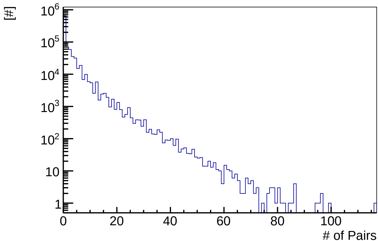
Step 5 : # of Valid Pairs
