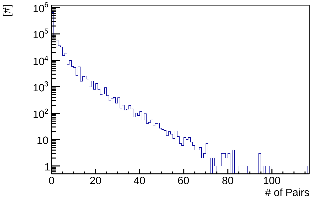
Step 4 : # of Valid Pairs
